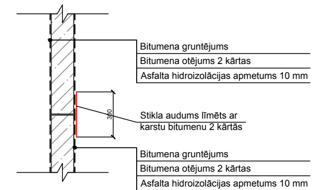
MEZGLS 2 1:10
