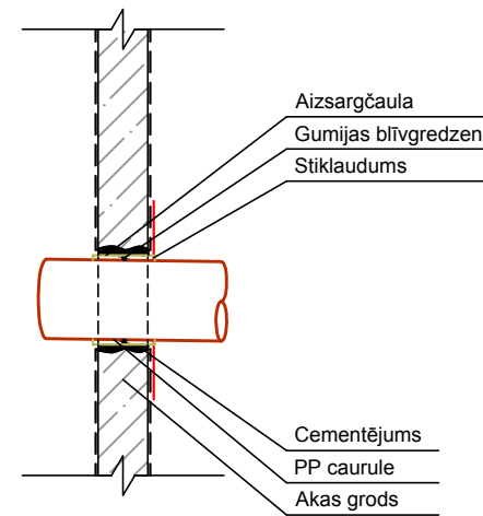
PP caurules ievads dz/b akā 1:10
