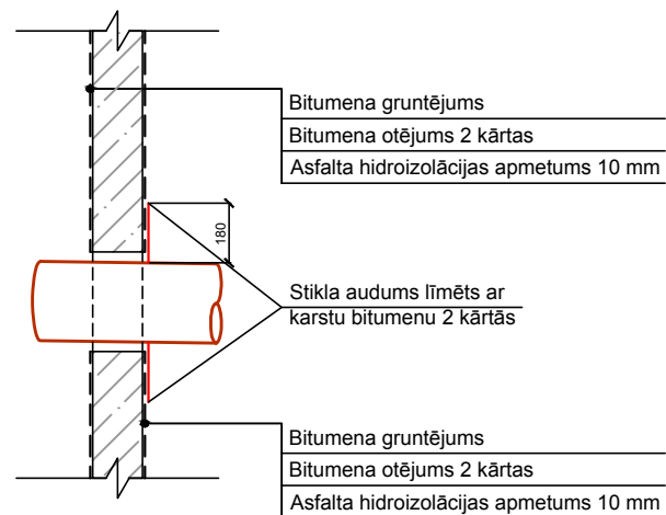
MEZGLS 1 1:10
