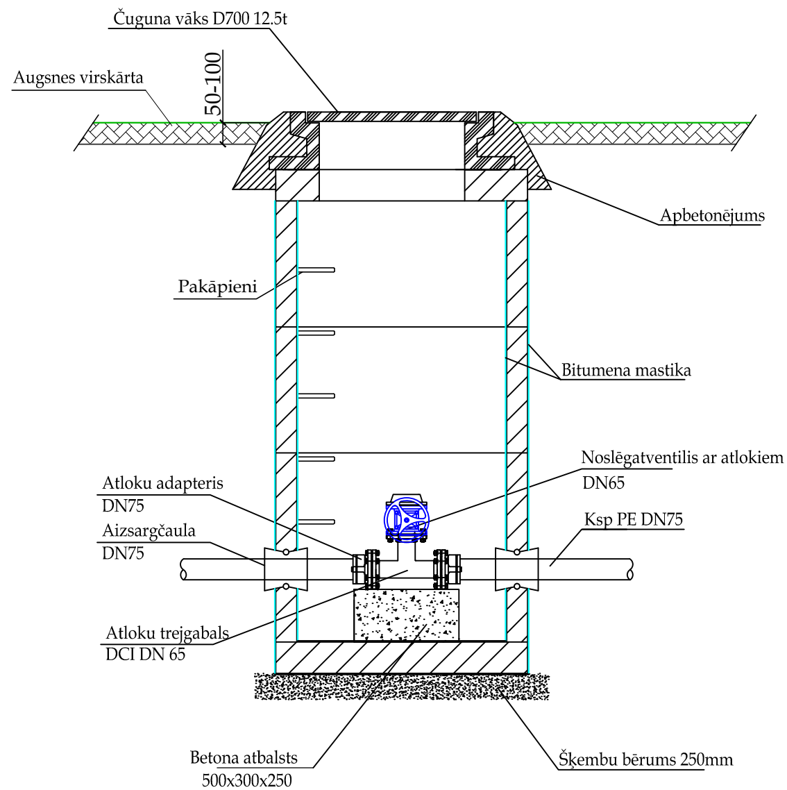
MEZGLS 1 1:10
