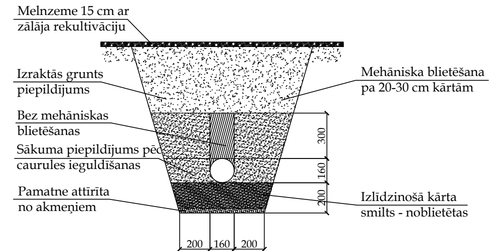
MEZGLS 2 1:10
